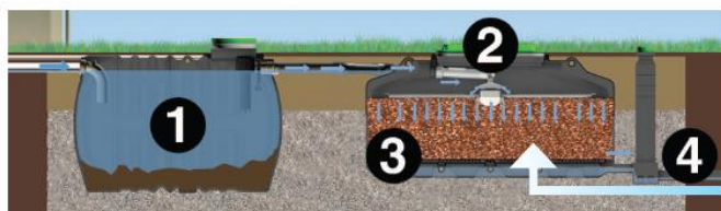
(1) Fossa com Pré Filtro (2) Filtro Compacto de Coco Premier Tech (3) Meio filtrante (fragmento de casca de coco) (4) Saida de efluente tratado
